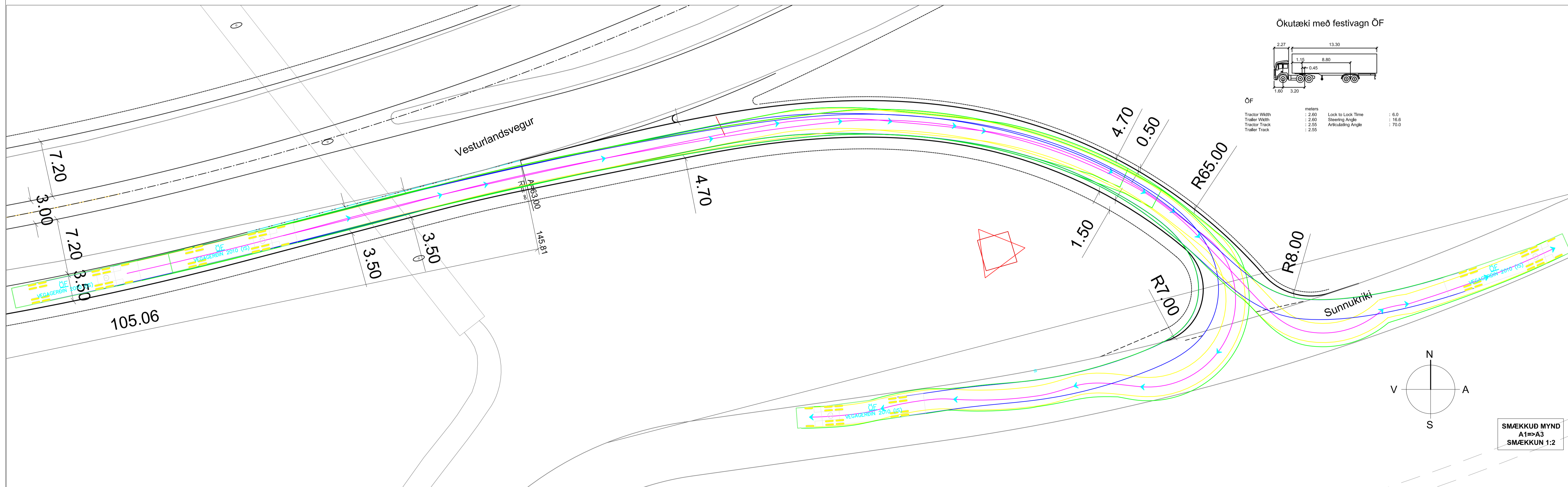
Grunnmynd 1:500
