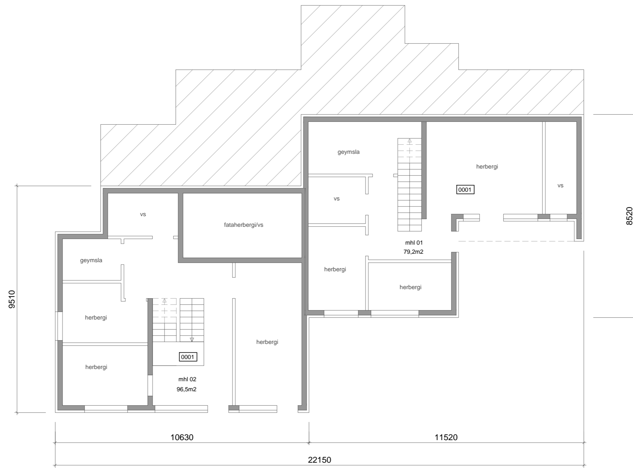
GRUNNMYND KJALLARA 1:100
