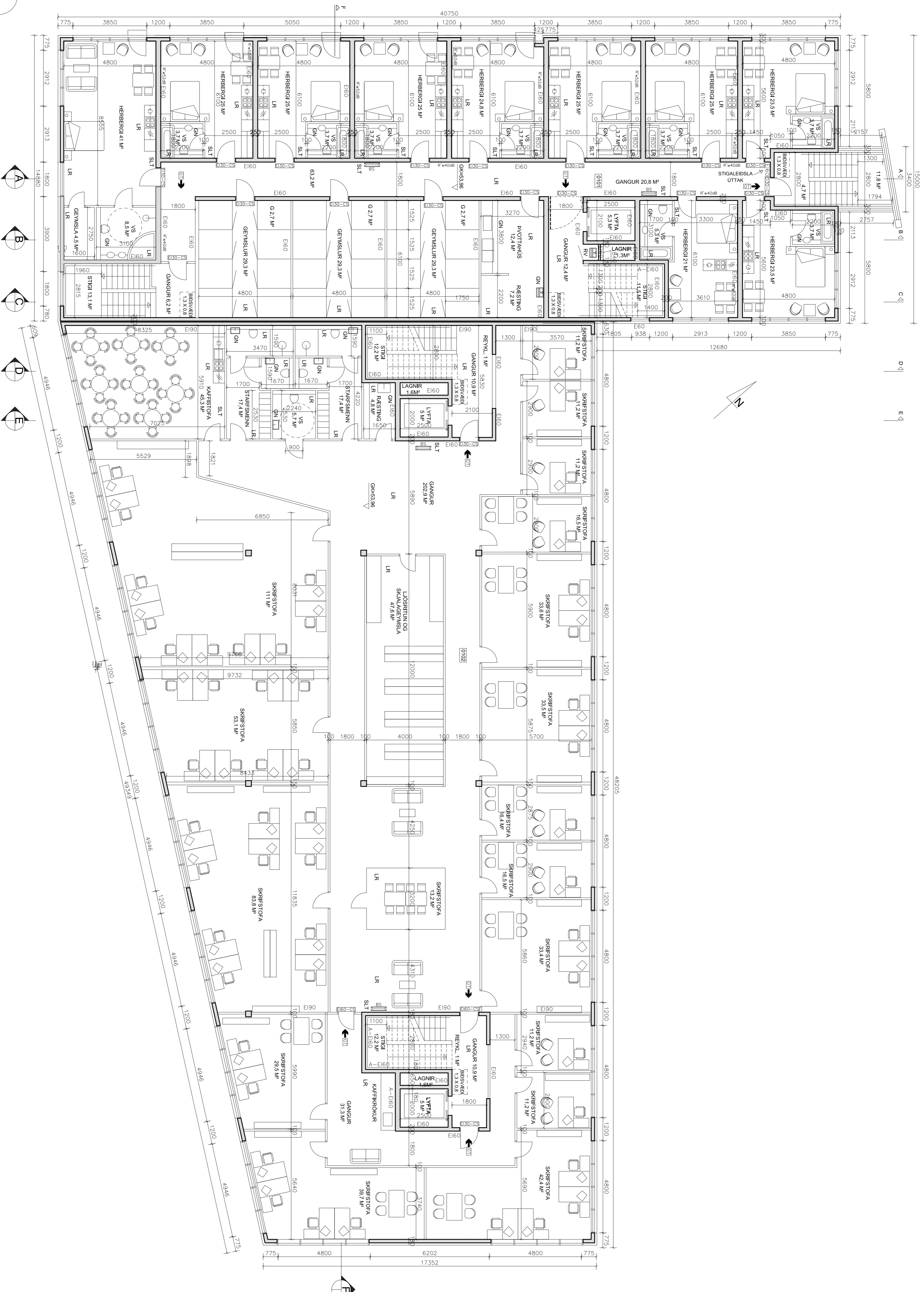
GRUNNMÝND 2.HÆÐ MKV. 1:100
