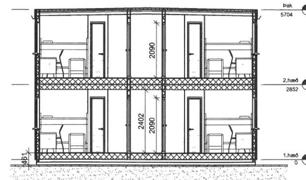
SNEIÐING
