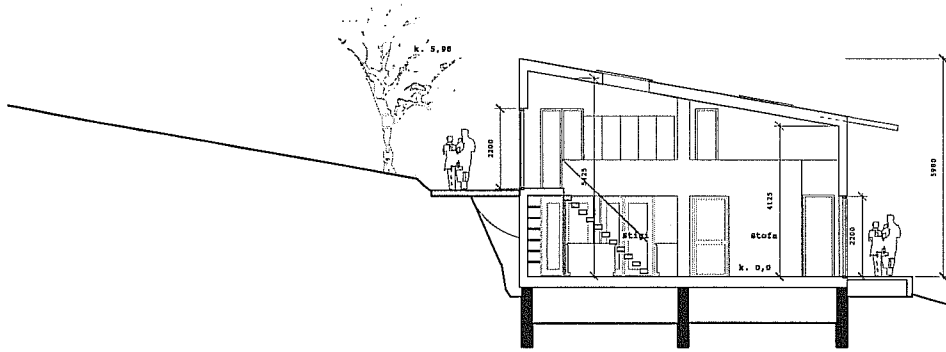
1 SNEIÐING 1 A2 - 02 1:100
