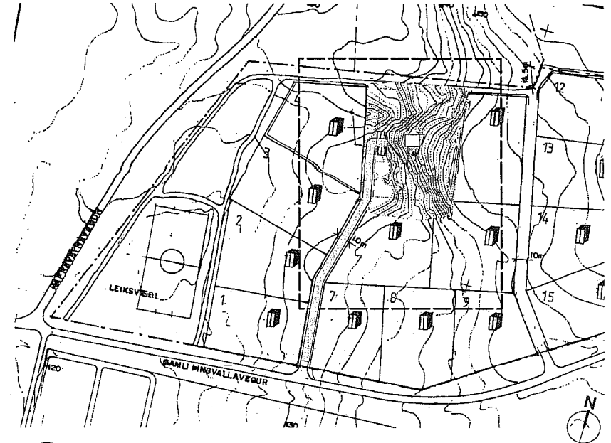
1 AFSTÖÐUMYND A2-01 1:2000
